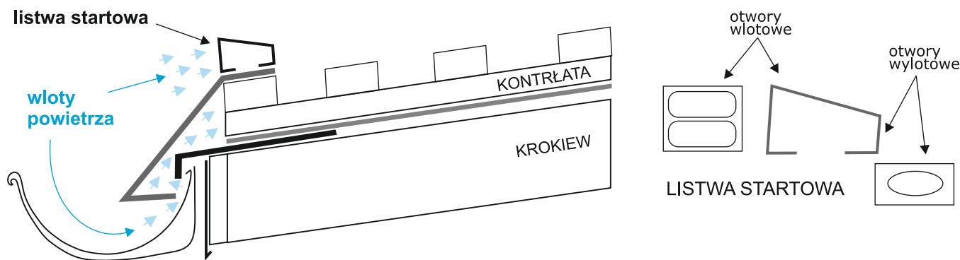
Rys. 5. Schemat montażu listwy startowej.
