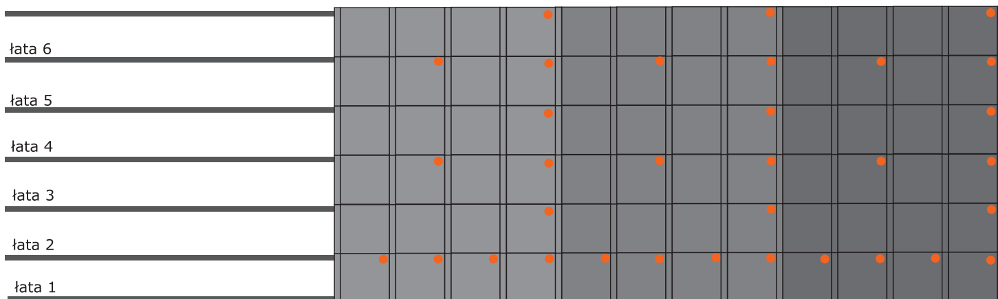
Rys. 7. Schemat rozmieszczenia wkrętów montażowych
